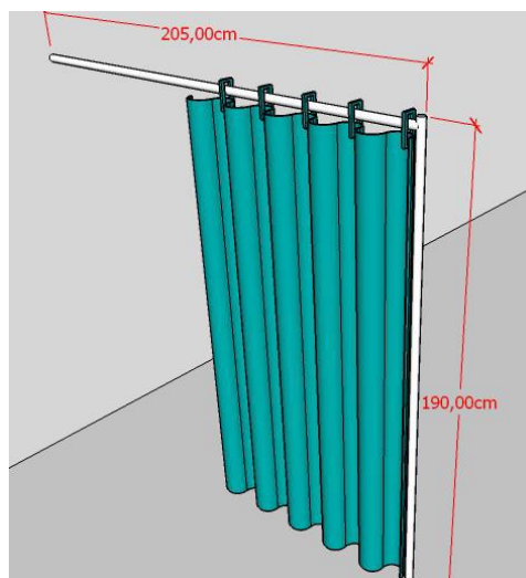
Figura 9 - Maquete eletrônica da proposta 4 – cortinas.
