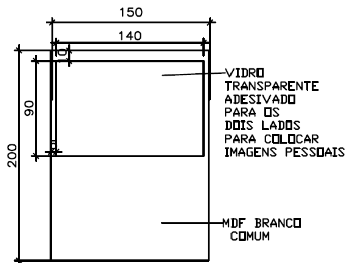
Figura 6: Vista cotada da proposta 2 – painel MDF.
